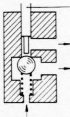
提動式方向閥，無內漏
