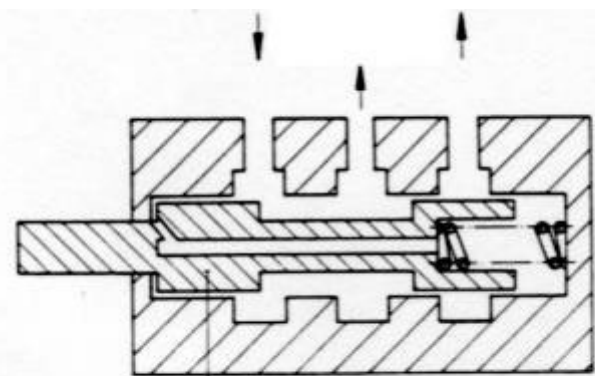
柱塞式方向閥，有內漏
