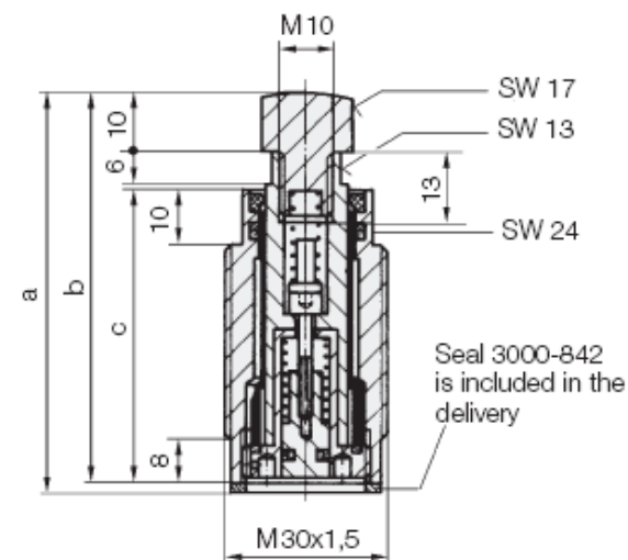
油壓頂出型
