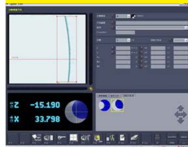
鑽石型體刀量測
