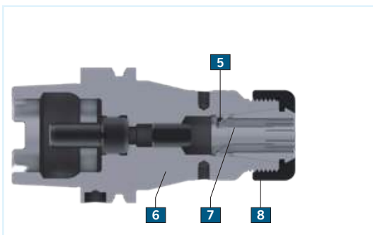
HAIMER強力型筒夾刀桿
