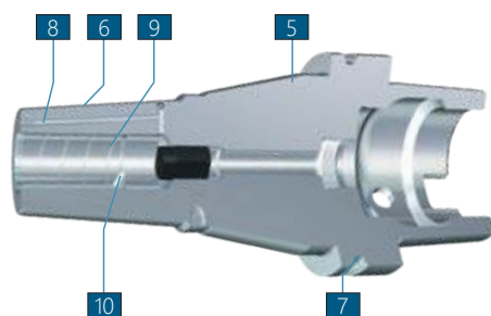
HAIMER 強力型燒結刀桿
