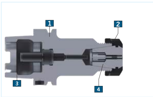
HAIMER 標準筒夾刀桿
