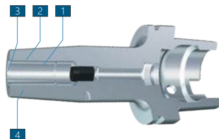
HAIMER 標準型燒結刀桿
