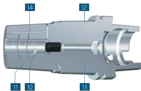
HAIMER 重型燒結刀桿
